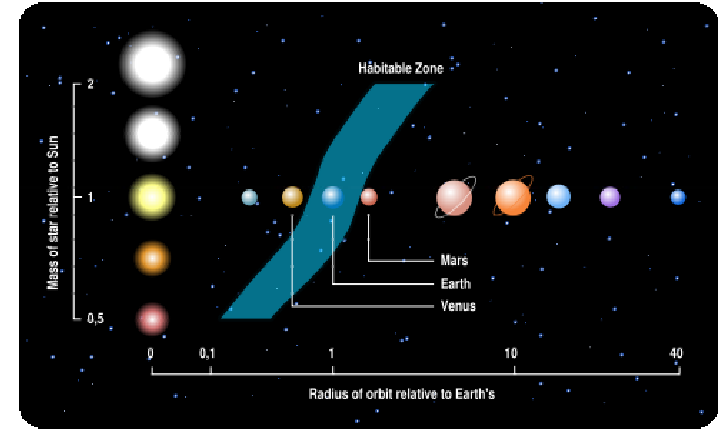
ISP209s8 Lecture 21
