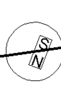
Uranus
