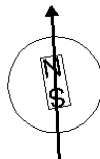
Jupiter
